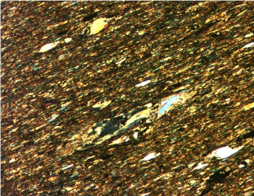
Bild 1: Ausschnitt aus der Probe Primero-Schiefer P15 (Schnitt senkrecht zur Schieferung), 100fache Vergrößerung, gekreuzte Polarisatoren, Aufnahme mit Texturanalysesystem
